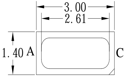
Fig. 1-2 SideView 侧面视图
